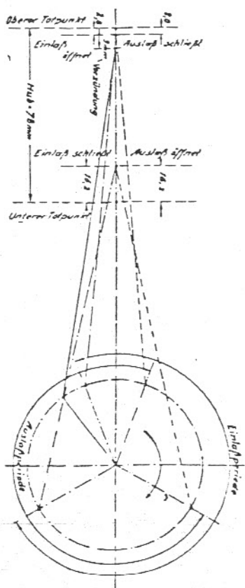
Abb. 27. Einstellprogramm für die Tourenmaschine
