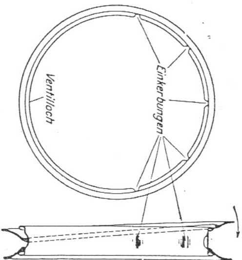
Abb. 32. Aufzeichnen von Drahtseilrissen auf Tiefbettsicherheitsfelgen
